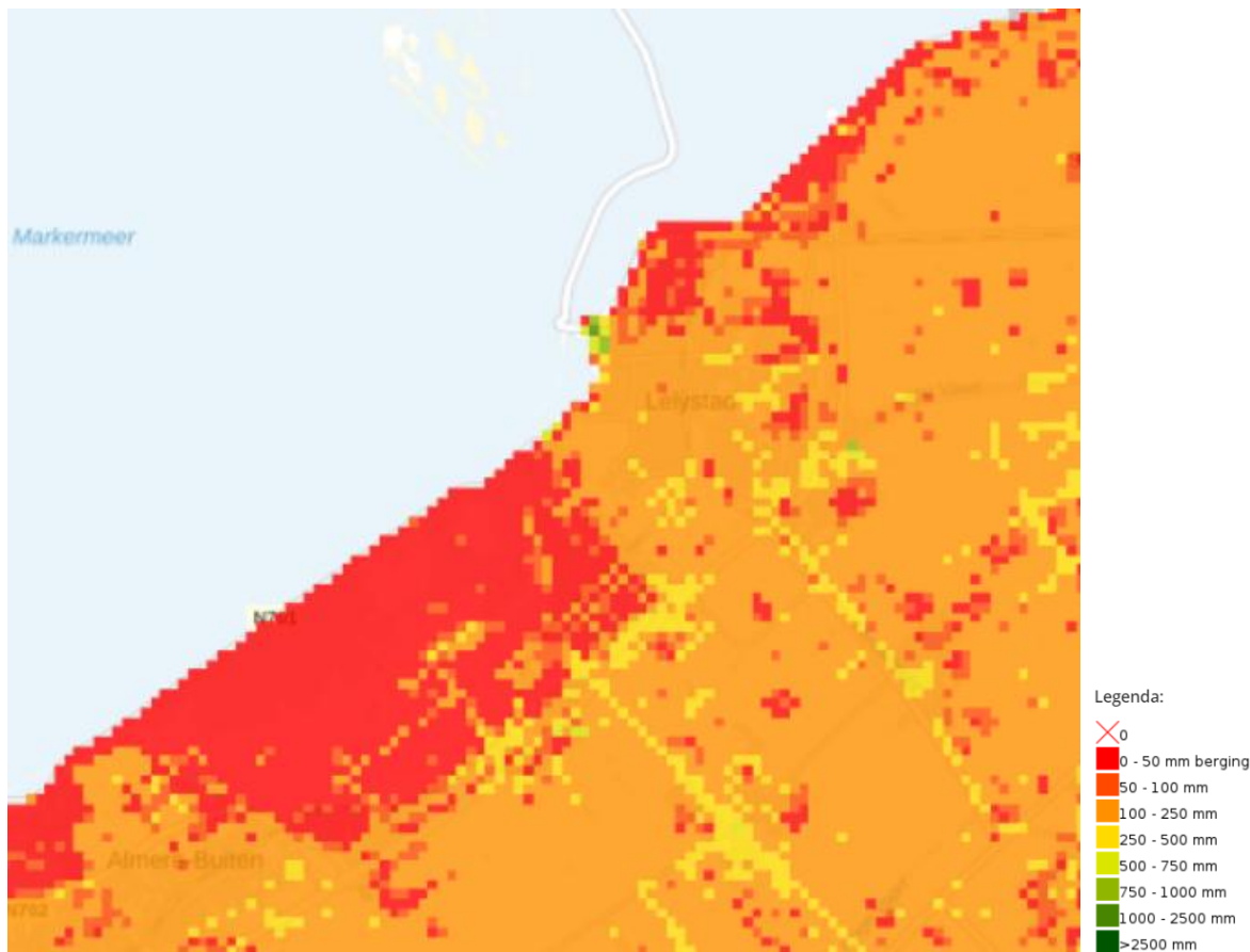
Figuur 4-19: Waterbergend vermogen van de ondergrond (Deltares, 2017).
