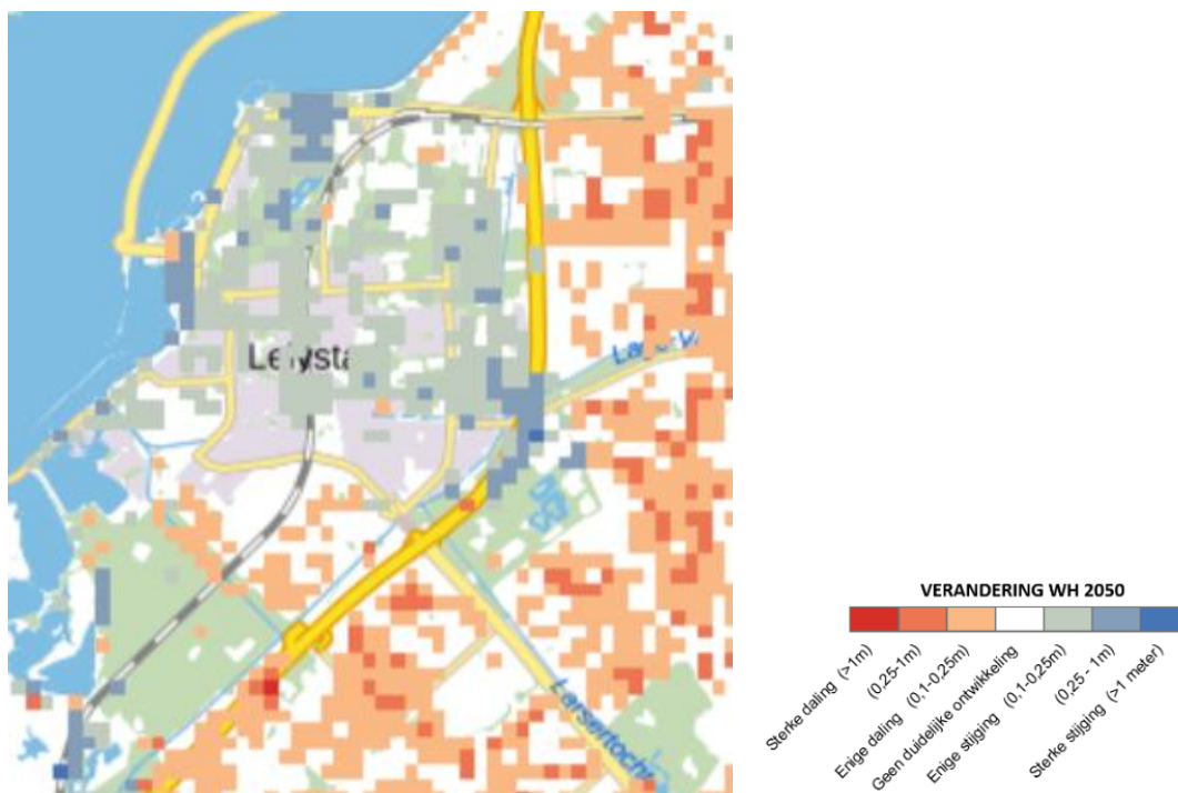
Figuur 4-24: Daling grondwaterstand in een extreem droge zomer, scenario 2050 hoog (Deltares, Nationaal Water Model, Klimaateffectatlas, 2019).
