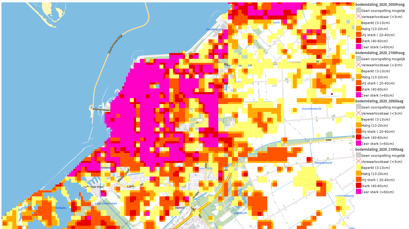
Figuur 4-6: Bodematlas Flevoland, bodemdaling voorspellingskaart tot 2100 – scenario hoog, sterke klimaatverandering.
