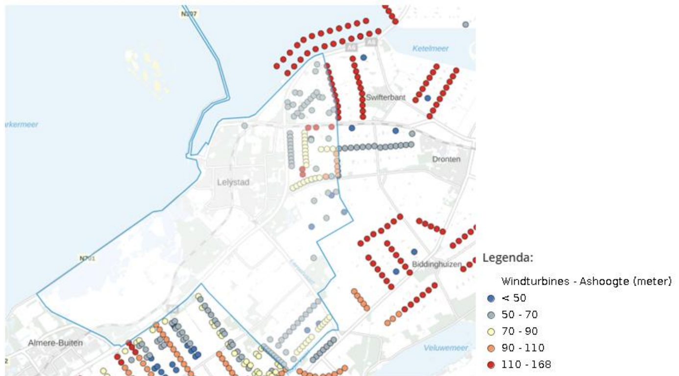
Figuur 4-60: Ashoogte Windturbines gemeente Lelystad
