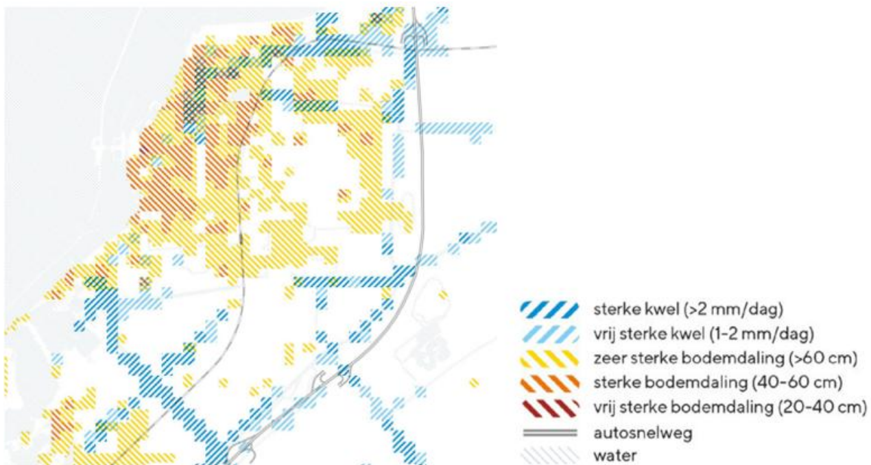
Figuur 4-5: Bodemkaart Lelystad, kwaliteitscatalogus (MUST, 2023).
